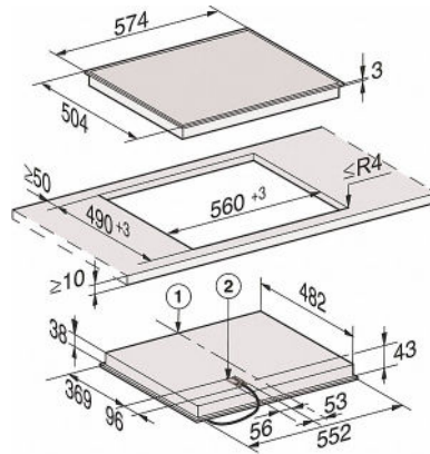
KM 6520 FR, KM 6538 FR (skitse)
